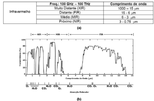
Fig. 4. a) Divisão da faixa do Infravermelho e b) Janelas de absorção de sinais infravermelhos da atmosfera.[5]
